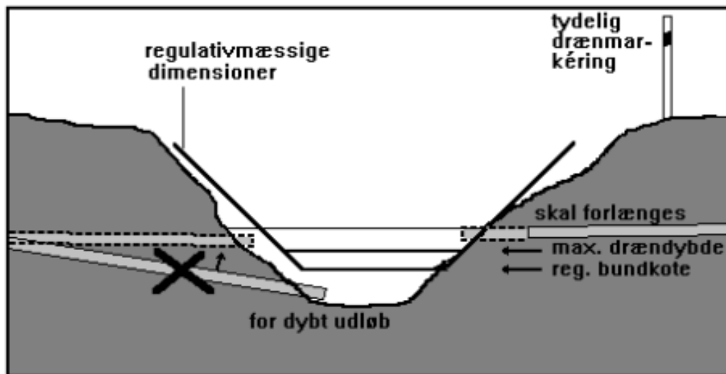
Forkert og korrekt anlagt drænudløb.
